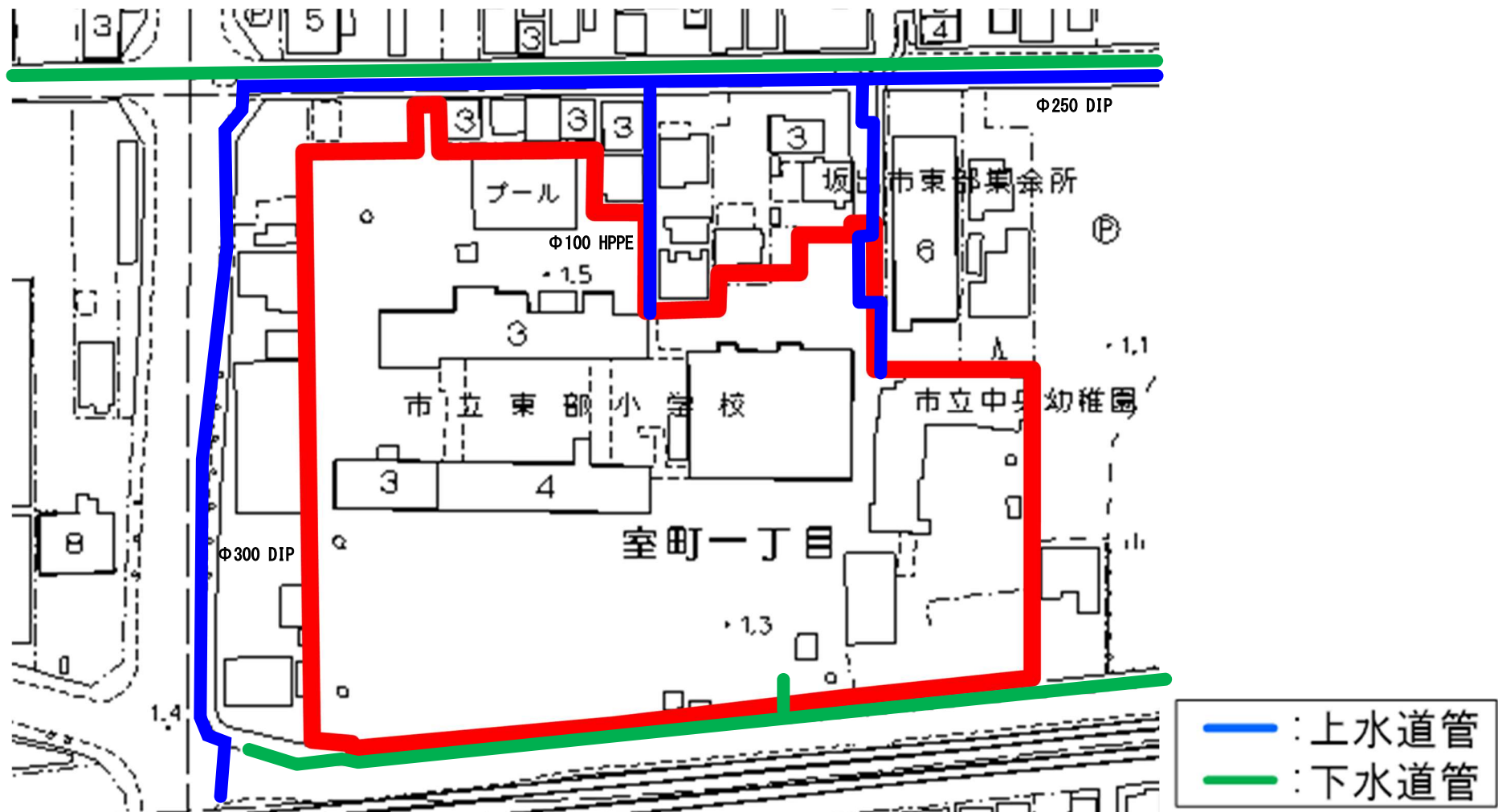
別紙資料1 「上水道・下水道参考図」
