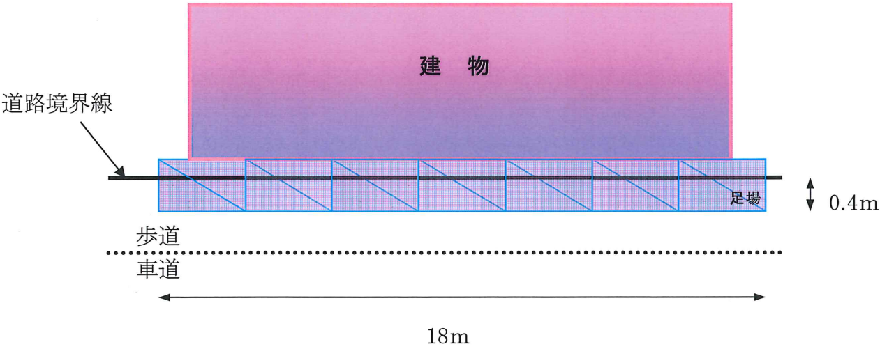
《平面図》
