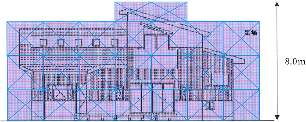
《立面図》
