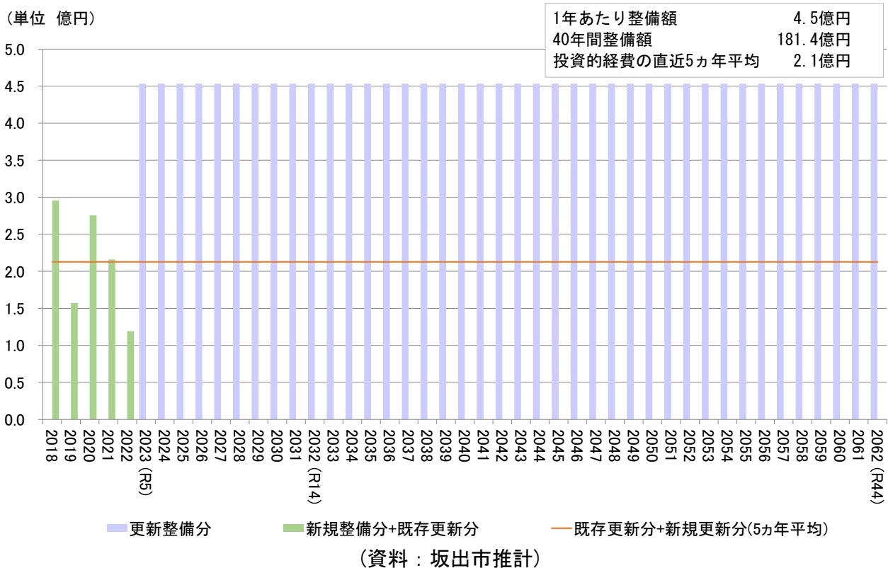
図表 6-8：港湾施設の更新費用予測
