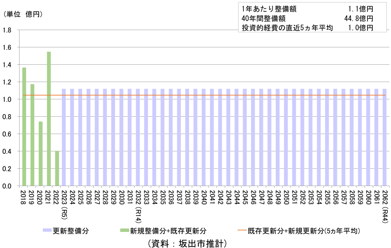
図表 6-11：漁港施設の更新費用予測
