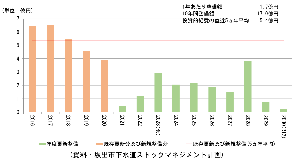
図表 7-2：下水道施設の更新費用予測
