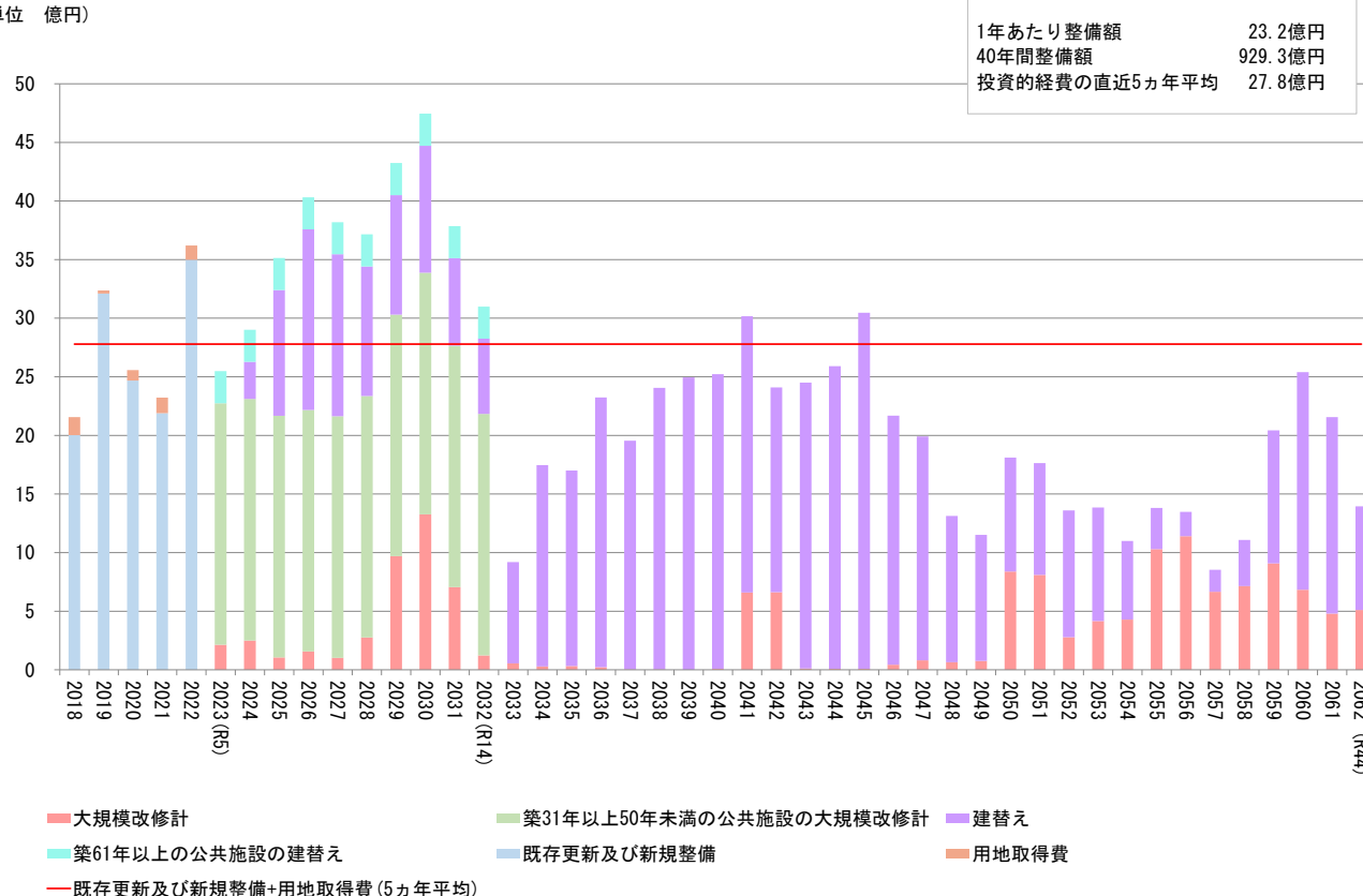
図表 3-5：建物系公共施設の更新費用 (現在保有している公共施設の全てをそのまま保有した場合)
