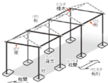
▲柱と柱の上に乗る「桁(けた)や梁(はり)」には一本の長い木材が必要
