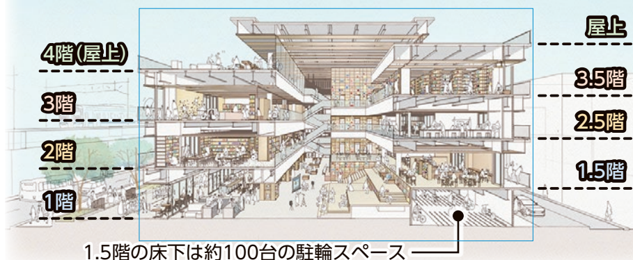
【駅前拠点施設の断面図】
