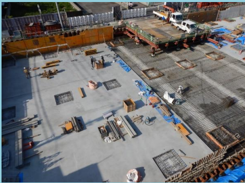
切梁を解体し、免震ピットの底が見えています。
